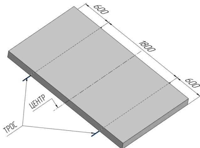
Рисунок 2 – Закладка тросов
