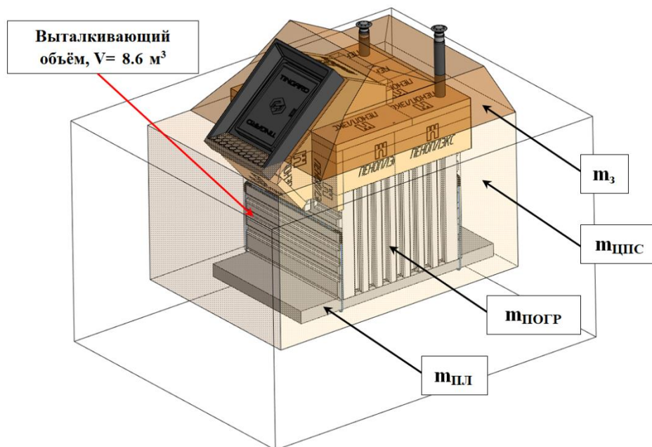
Рисунок 13 – Расчет якорения погреба
